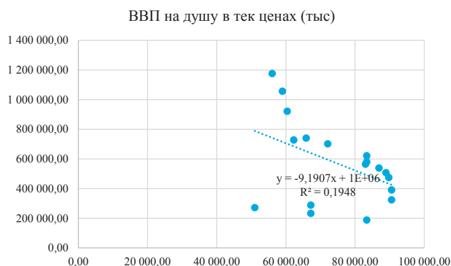
Рис. 1. Корреляционное поле количества СМИ от ВВП с линией тренда
