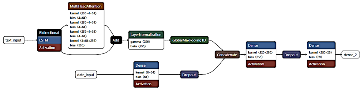
Рис. 4. Архитектура нейронной сети для sentiment-анализа новостных постов в Telegram на данных канала «Топор Live». Составлено авторами с помощью сервиса Netron [2]
